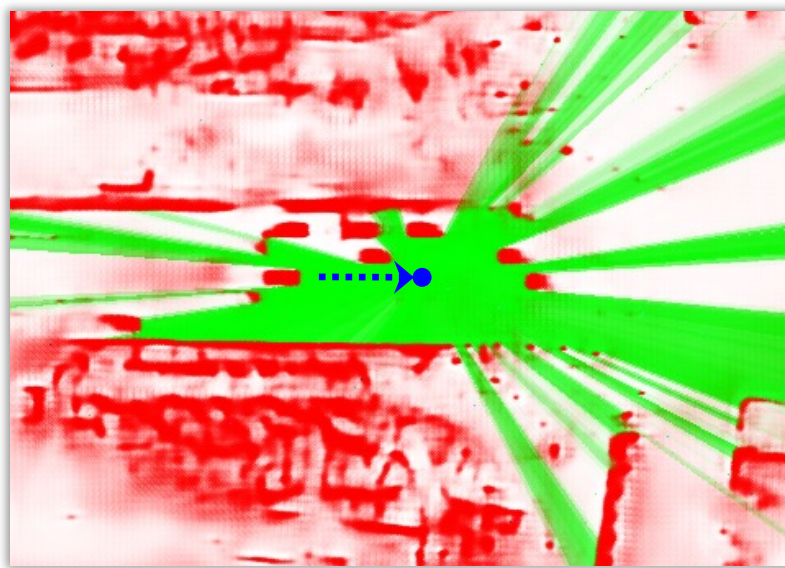
(b) New sensor position y + \Delta y , Scene s
